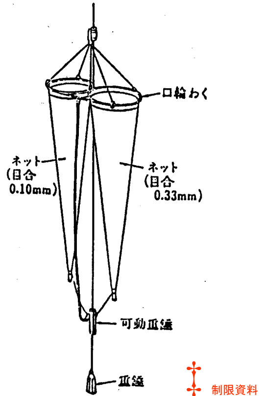
図 4.1 並列型 NORPAC ネットの例 (Motoda, S. 1957. North Pacific standard plankton net. 日本プランクトン研究連絡会報 第4号より引用)
