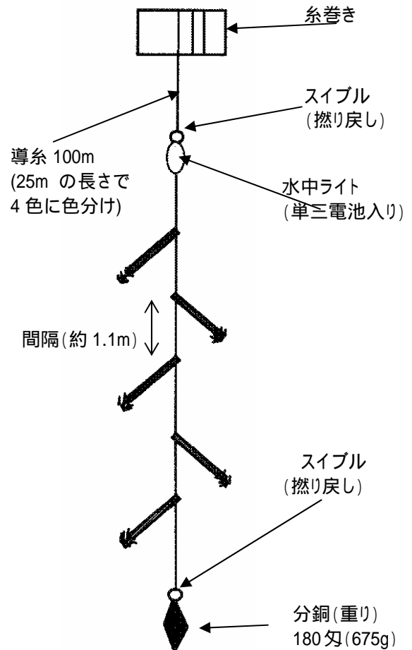
図 5.1 イカ釣り具の構成
