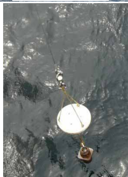
図 2.3 透明度板による濁度計
