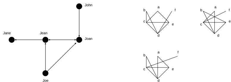
図 10: John, Joan, Jean, Jane 及び Joe の関係図 (左). 考え得る対戦カードを表す 5 種類のグラフ (右).
