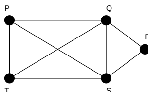
図 1: この講義で扱う「グラフ」の一例。このグラフの点数は n = 5 、辺数は m = 8 であり、それぞれの点の次数は \deg(P) = \deg(T) = 3 , \deg(Q) = \deg(S) = 4 , \deg(R) = 2 である。
