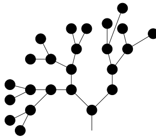
図 7: 木の一例.
