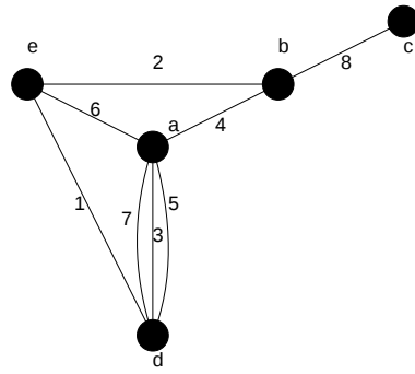
図 21: 隣接行列が で与えられるグラフ. ここで, 接続行列 の第 1 列, 2 列 ... の番号として, 図の a,b, ... が対応していることに注意.
