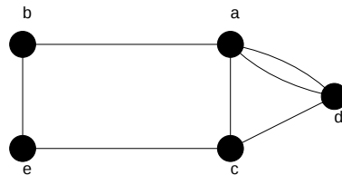
図 20: 隣接行列が で与えられるグラフ. ここで, 隣接行列 の第 1 行, 2 行, ... の番号として, 図の点 a, b, ... が対応していることに注意.
