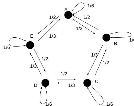
図 198: 遷移行列 P に対応する有向グラフ.
